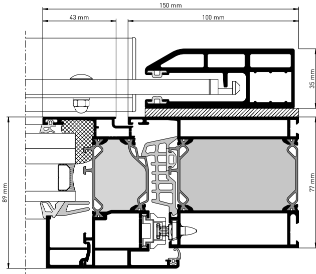
heroal W 77 + Rolladen heroal RS 37 RC 3
