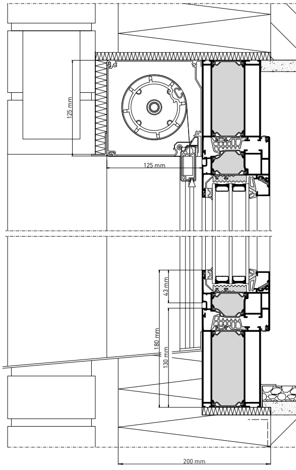
heroal W 77 PH mit Sonnenschutzsystem VS Z
