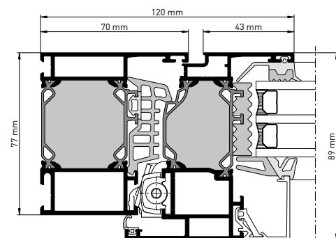
heroal W 77 mit Beschlagsystem heroal WF 100 i
