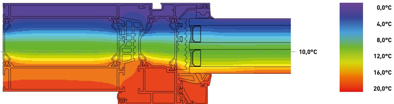
Isothermenverlauf nach U_i EN ISO 10077-2
