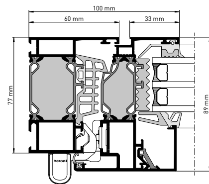
heroal W 77 mit Beschlagsystem heroal WF 100
