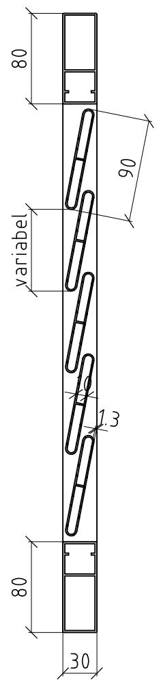
Schnitt A-A
